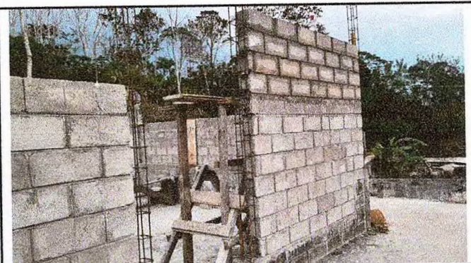
Foto 4: Avance de un 55% de las paredes de los dos módulos.
