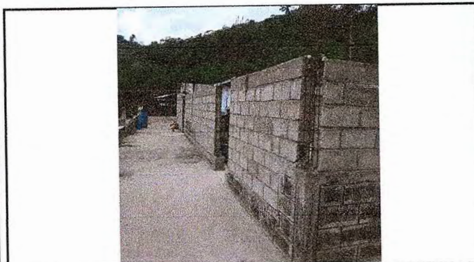
Foto 3: Vista del corredor de los dos módulos con blocks colocados en un 50%.
